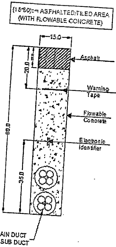
حفرية بايمنت سم 15 سم 60 مأسورة عدد 2 في مناطق اعادة وضع اسفلت / بلاط
