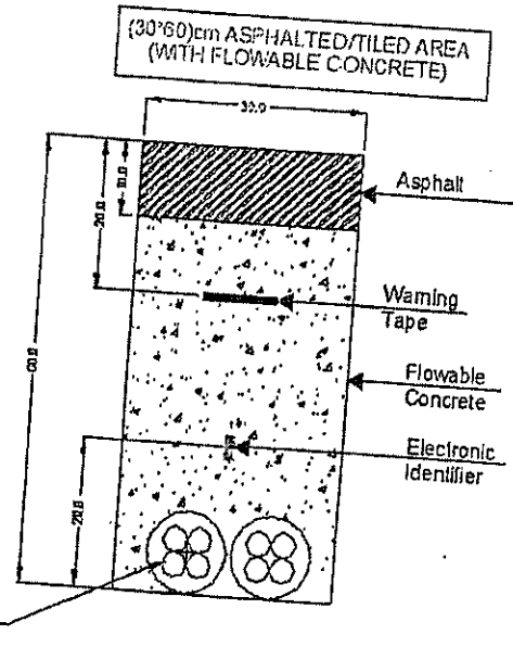
حفرية بايمنت سم 30 سم 60 مأسورة عدد 2 في مناطق اعادة وضع اسفلت / بلاط
