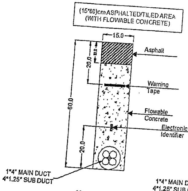
حفرية بايمنت سم 15 سم 60 مأسورة عدد 1 في مناطق اعادة وضع اسفلت / بلاط
